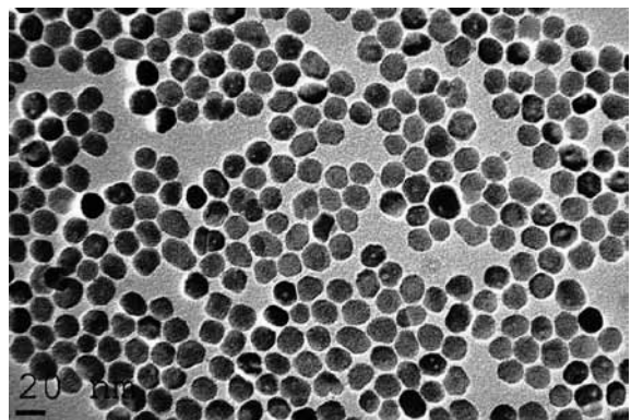
Slika 1: Magnetni nanodelci
