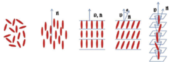
Slika 4: Skica tekočokristalnih faz: izotropna, nematska (N), smektična A ( \text{SmA} ), smektična C ( \text{SmC} ) in feroelektrična smektična \text{C}^* ( \text{SmC}^* )
